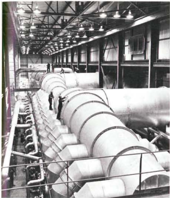
Des monteurs mettent la dernière main aux fours d'une nouvelle usine de boulettage à Atikokan, située à l'ouest de Port Arthur (Ont.). À la suite des vastes programmes d'expansion dans la production du minerai de fer au cours des dernières années une tendance se dessine vers l'agglomération d'une plus forte proportion de la production actuelle, augmentant ainsi brusquement le rapport boulettes-minerais.
